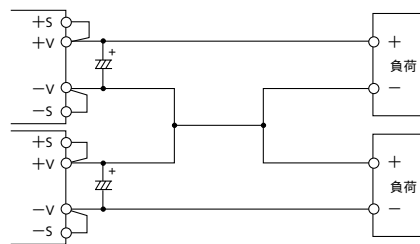
図12-2 ±出力使用の直列運転
