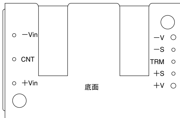
入出力端子配列 (底面より)
