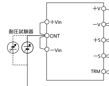
図19-1 入力-出力間耐電圧試験方法
