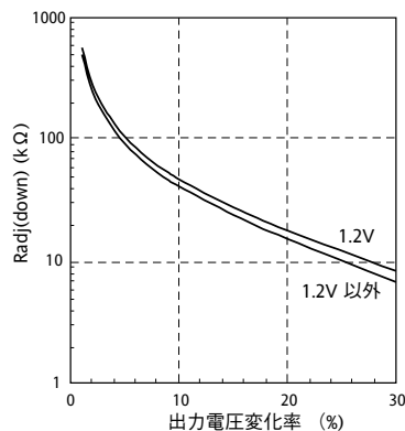
図2-3 △(%) 対外付け抵抗(1)
