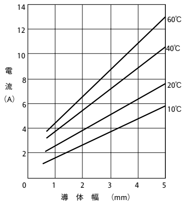
図2-2 銅箔35 \mu mに於ける容量電流対導体幅特性
