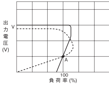
——— : 電源負荷特性 - - - - - : 負荷側特性(ランプ、モーター、定電流負荷など) 注) ランプ、モーター、定電流負荷などの場合、A点で立上がり荷が停止することがあります。
